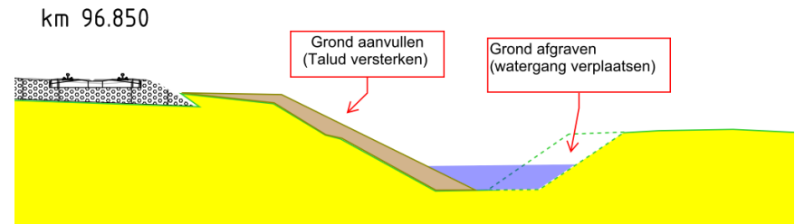
Nieuwe situatie
