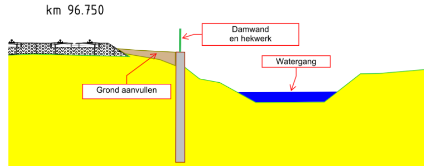
Nieuwe situatie
