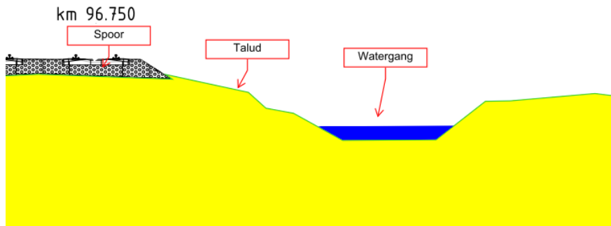
Bestaande situatie
