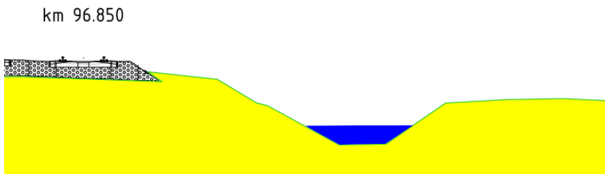
Bestaande situatie
